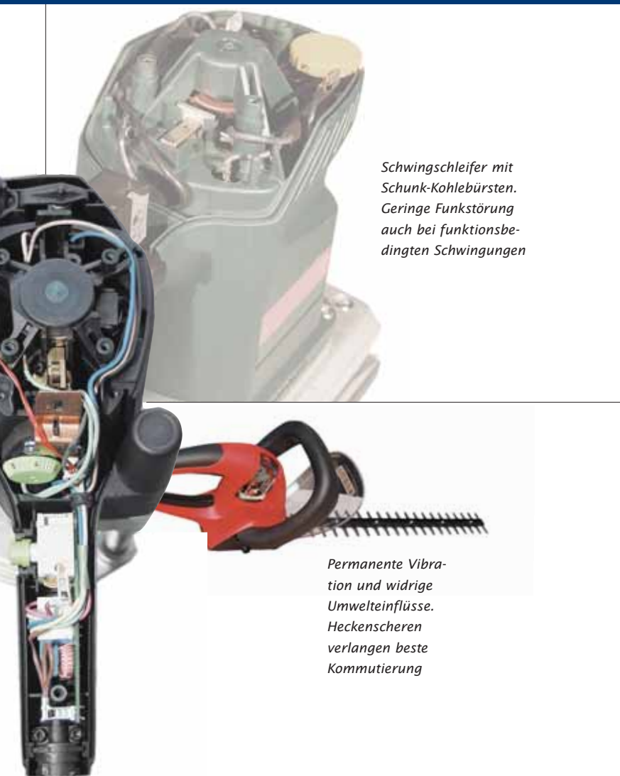
Für extreme Belastungen. Kohlebürsten mit besonderer Schonung des Kommutators
